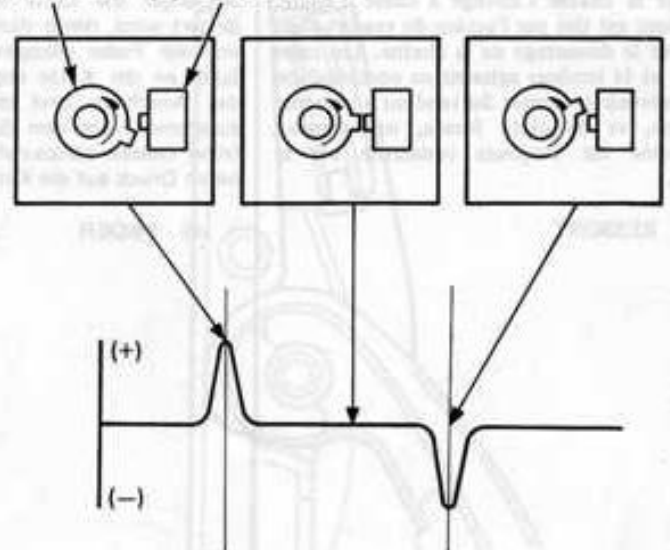
(1) ROTOR (2) GENERATOR
